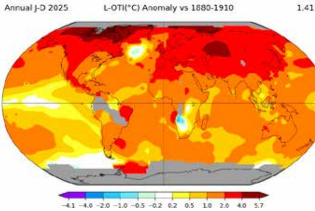
Abbildung 1: Die Karte zeigt die Temperaturabweichungen im Jahr 2025 verglichen mit der durchschnittlichen Temperatur im Zeitraum 1880-1910. [1]
